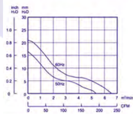
Curva de rendimiento del ventilador
