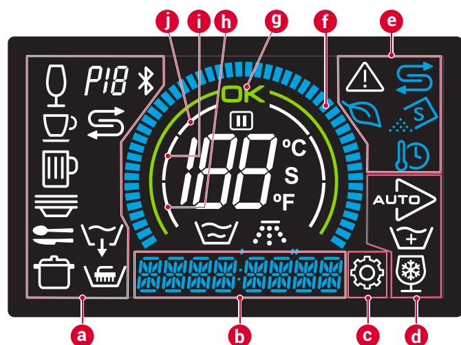
Fig. 3: Pantalla LCD
