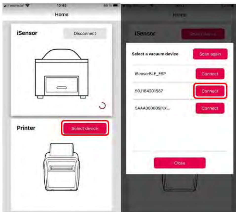
Figura 18. Selección y sincronización de la impresora
