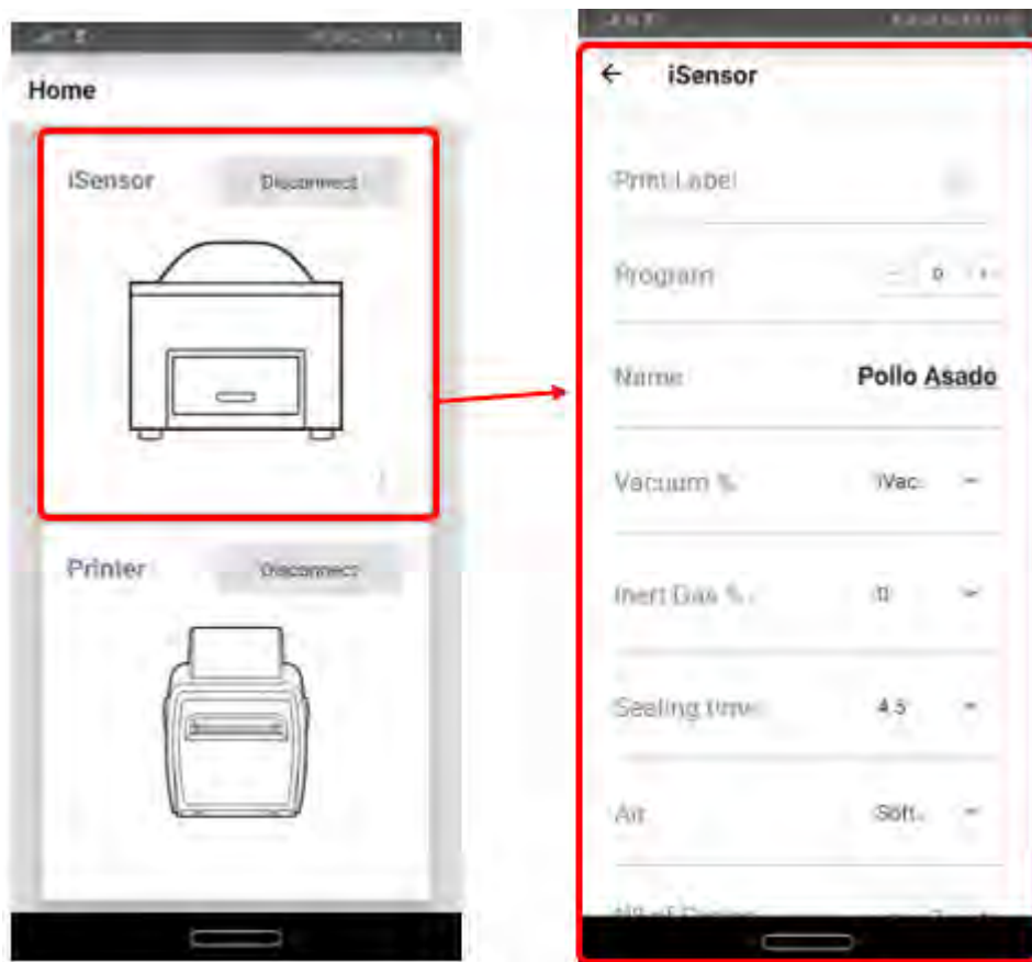
Figura 20. Edición de programas iSensor
