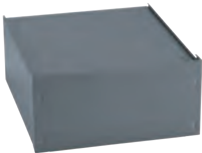
APWM 037 Zócalo cerrado de 30 cm de altura para la carga y descarga ergonómica de las lavadoras. • Al/An/Fo: 30,00 cm – 69,80 cm – 79,20 cm
