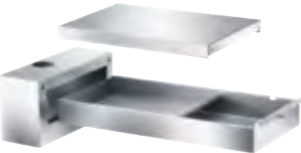
APCL 021 Cajón del filtro de pelusas de acero inoxidable para filtrar las pelusas y las partículas gruesas del agua de lavado. • Para la instalación en un zócalo adecuado • Fácil extracción para una limpieza rápida y sin complicaciones. • Filtro de pelusas en acero inoxidable, se extrae con facilidad • Volumen 24 litros • Diámetro de racor de empalme hacia atrás de 70 mm • Al/An/Fo: 25,00 cm – 49,85 cm – 86,00 cm
