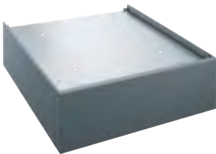
APWM 021 Zócalo cerrado de 30 cm de altura para la carga y descarga ergonómica de las lavadoras. • Al/An/Fo: 29,00 cm – 78,50 cm – 89,50 cm
