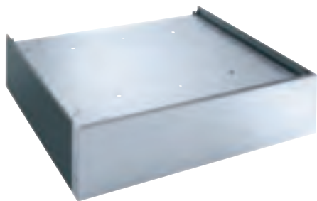
APWM 031 Zócalo cerrado de 25 cm de altura para la carga y descarga ergonómica de las lavadoras. • Al/An/Fo: 25,50 cm – 92,00 cm – 85,50 cm
