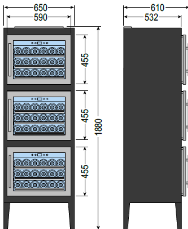
VINITY 3 V (MEDIDAS)
