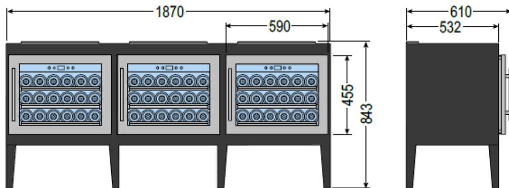
VINITY 3 H (MEDIDAS)
