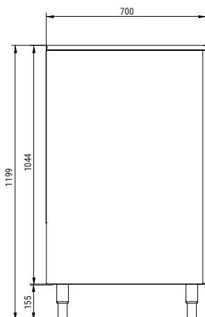
LEFT SIDE VIEW VISTA LATERAL IZQUIERDA
