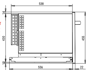
RIGHT SIDE VIEW VISTA LATERAL DERECHA
