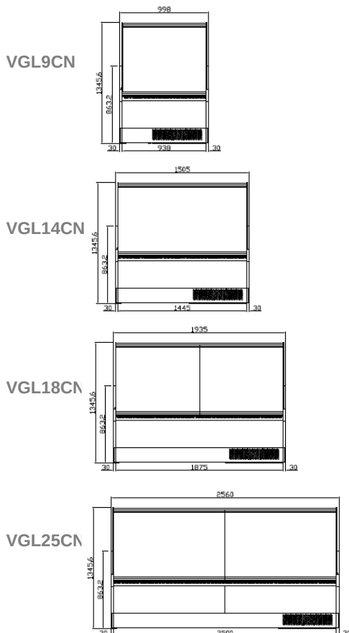
ALZADO
