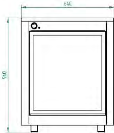
ALZADO
