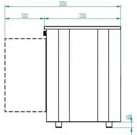
PERFIL
