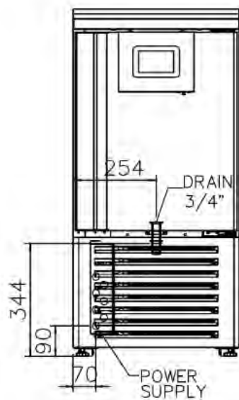
ALZADO
