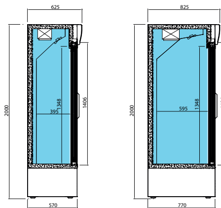
ERC 65
