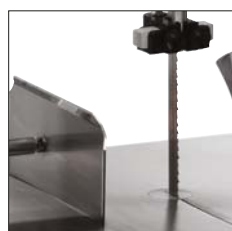
Regulación espesor y altura de corte. freno motor. Superficie de trabajo y guía cuchilla de acero inox.
