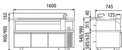
Modelo MCR-160D
