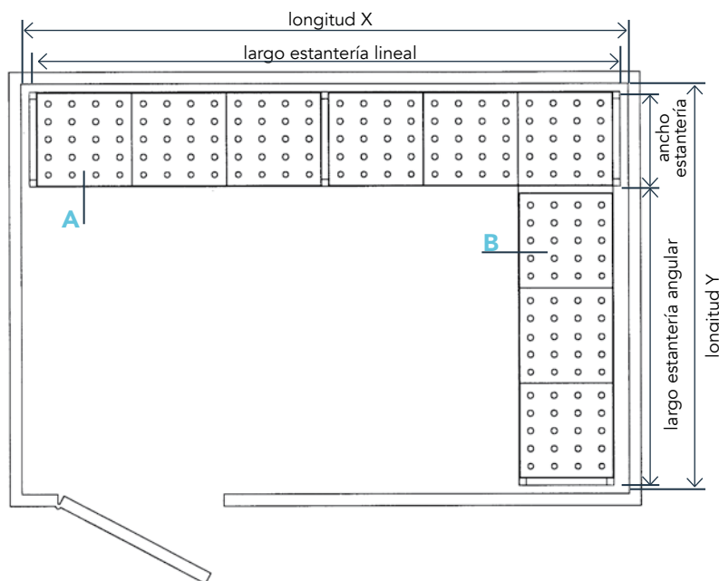
A-estantería lineal
