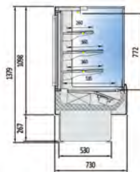
VSSA-6-6-R VSSA-6-9-R VSSA-6-13-R
