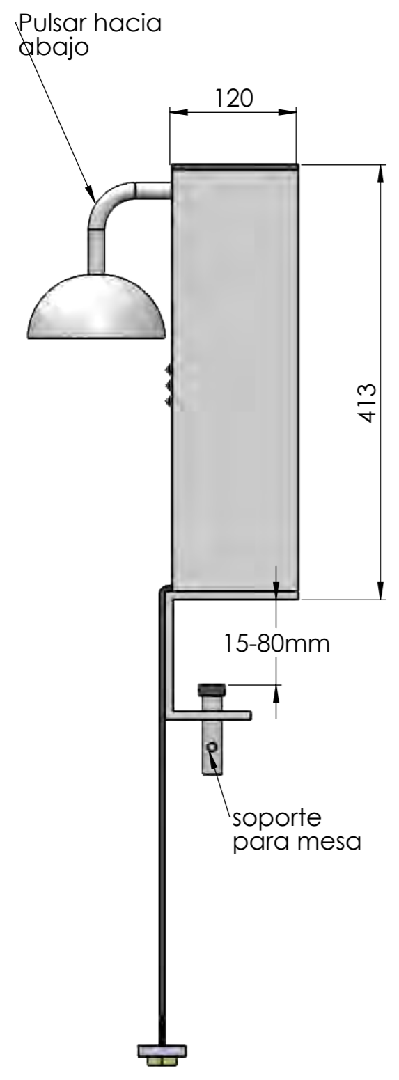
ALZADO
