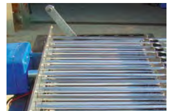
Estante giratorio para espeto (230V) Rotating skewer with motor (230V)
