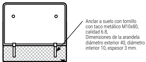
SECCIÓN D-D
