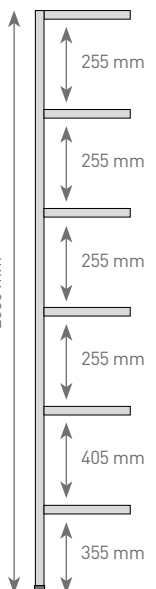
Altura 2050 mm / 6 niveles Height 2050 mm / 6 levels Hauteur 2050 mm / 6 niveaux Höhe 2050 mm / 6 Ebenen
