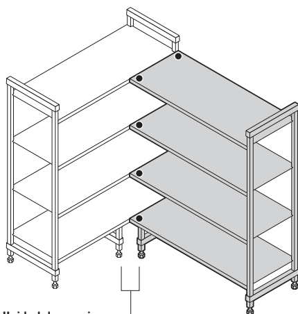
Unidad de esquina base + unidad suplementaria usando 1 juego de conectores de esquina por estante y 2 soportes de estiba.
