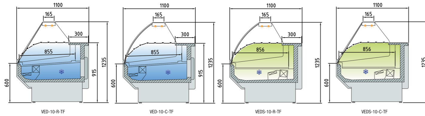
MODELOS CON RESERVA / RESERVE MODELS / RÉSERVE MODÈLES
