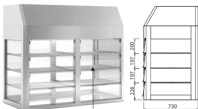
Estante de metacrilato opcional Shelf methacrylate optional Étagère vitrée en option
